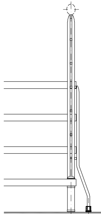
Irrigidimento montante rampa ESTERNO
