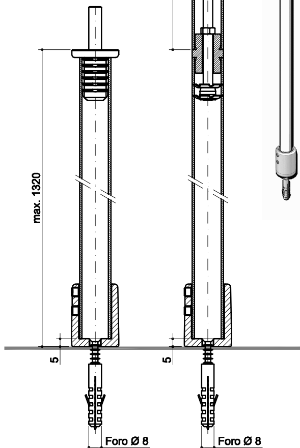
Esempio di piede a terra singolo
